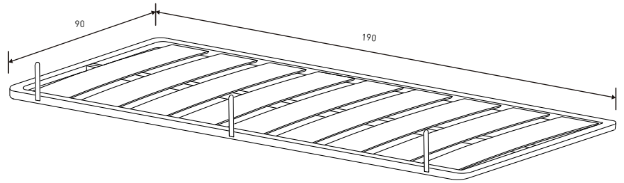
SOMIER ARRASTRE 3 PLETINAS 24,96 puntos
