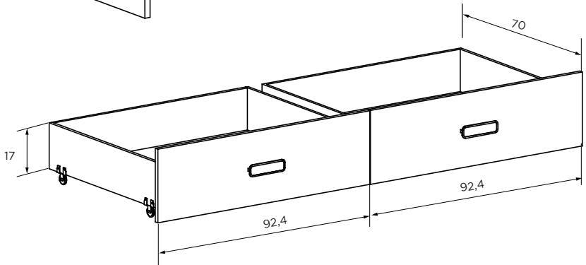
CAMA COMPACTO CON CAJONERA 149,35 puntos Cambria-blanco
