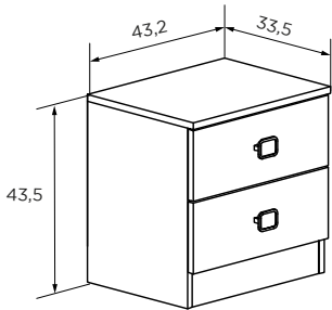
MESITA DE NOCHE 23,35 puntos Cambria-blanco
