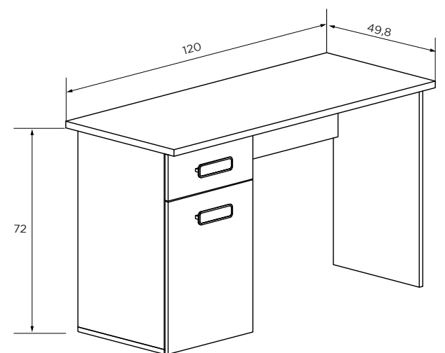
MESA ESTUDIO 46,30 puntos Cambria-blanco
