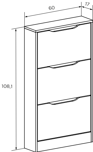
ZAPATERO 3 PUERTAS 36,20 puntos Cambria- blanco
