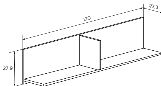
ESTANTE L 120 CM. 15,05 puntos Cambria-blanco
