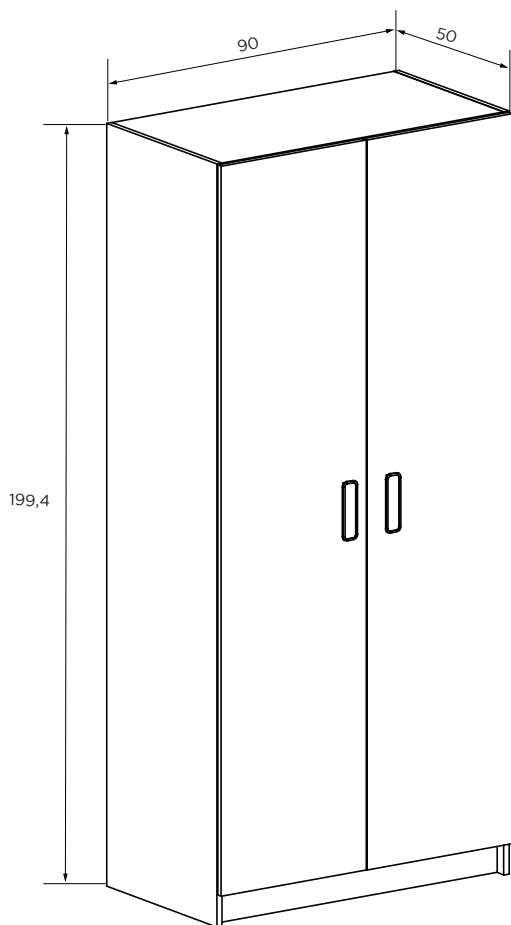
ARMARIO 2 PUERTAS 90 puntos Cambria-blanco Incluye 1 estante y 1 barra para colgar.
