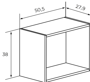
ESTANTERÍA CUBO 15,45 puntos Cambria
